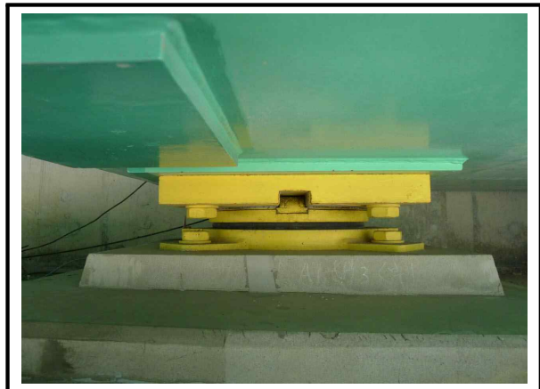
사진번호 10 교량받침 전경 외관망도 -
