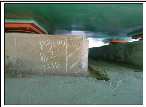
사진번호 37 교량받침 P3 Br2(A2) 외관망도 53-1 콘크리트 들뜸
