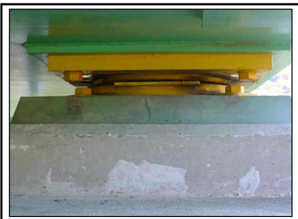
사진번호 39 교량받침 P5 Br6 몰탈 외관망도 55-1 균열(0.3mm 미만)
