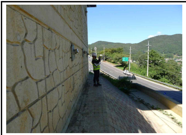
사진번호 57 도보로 하부(교대) 외관조사현황 외관망도 -
