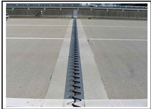
사진번호 8 신축이음 전경 외관망도 -
