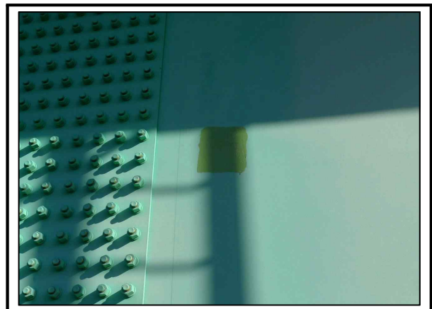
사진번호 30 거더외부 S2 G3 RW 보수현황 외관망도 -
