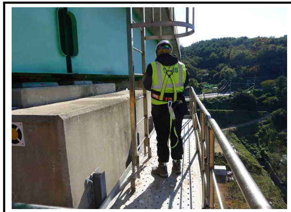
사진번호 58 교량점검시설을 이용한 외관조사현황 외관망도 -
