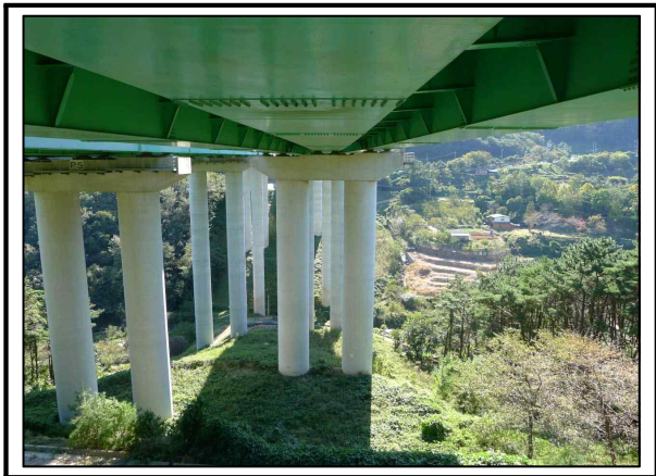
사진번호 50 교각 P5 기초 매립 외관망도 -
